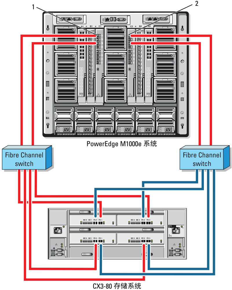
图 2-11. 具有嵌入式光纤信道交换机模块的外部网络连接群集
